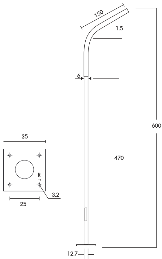
PT-04/6-1/LN เสาเทเปอร์ทั้งตัวยาว 2.00" สูง 6.00m.
