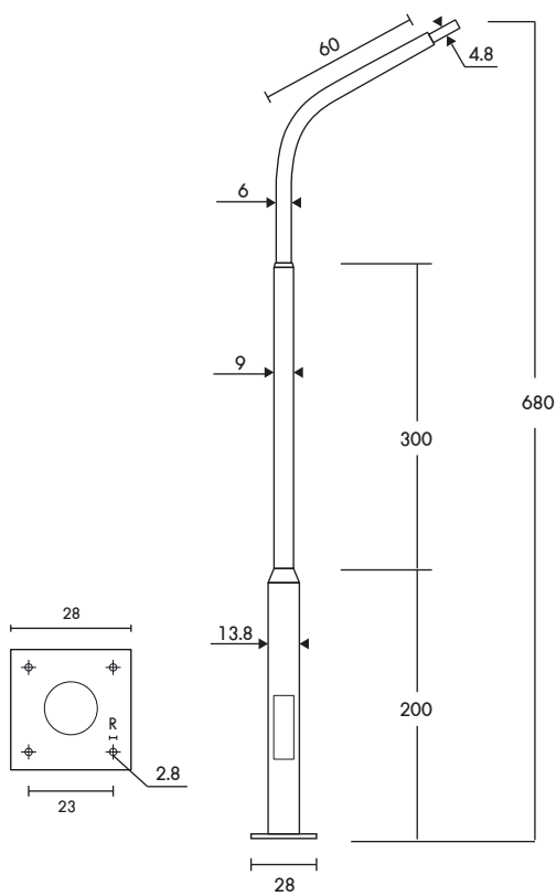
PT-03/7-1/15 ราคา 16,600.- เสาถึงเดี่ยวปลาย 1.50" สูง 7.00m.
