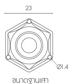
PT-A5-5007/2 E27 x 2 Aluminium Color Black ■ 6,720.- *ราคารวมเสา
