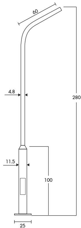
PT-03/3-1/15 ราคา 5,830.- เสาถึงเตี้ยวปลาย 1.50" สูง 3.00m.
