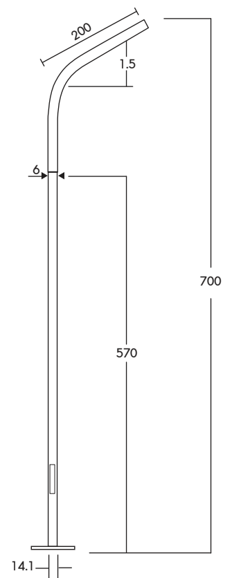
PT-04/7-1/VJ เสาเทเปอร์ทั้งตัวยาว 2.00" สูง 7.00m.
