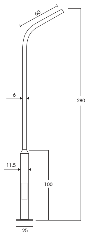
PT-03/3-1/20 ราคา 6,270.- เสาถึงเตี้ยวคู่ปลาย 2.00" สูง 3.00m.
