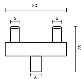
PT-06-A2 ตัวหลอด 2 หัว 1,800.-
