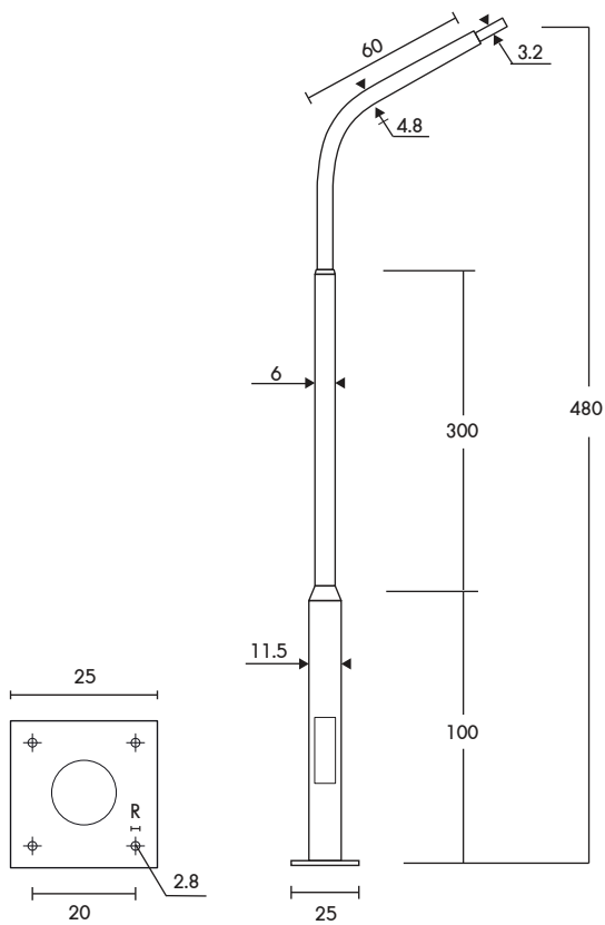
PT-03/5-1/10 ราคา 8,960.- เสาทั้งตัวยาวปลาย 1.00" สูง 5.00m.
