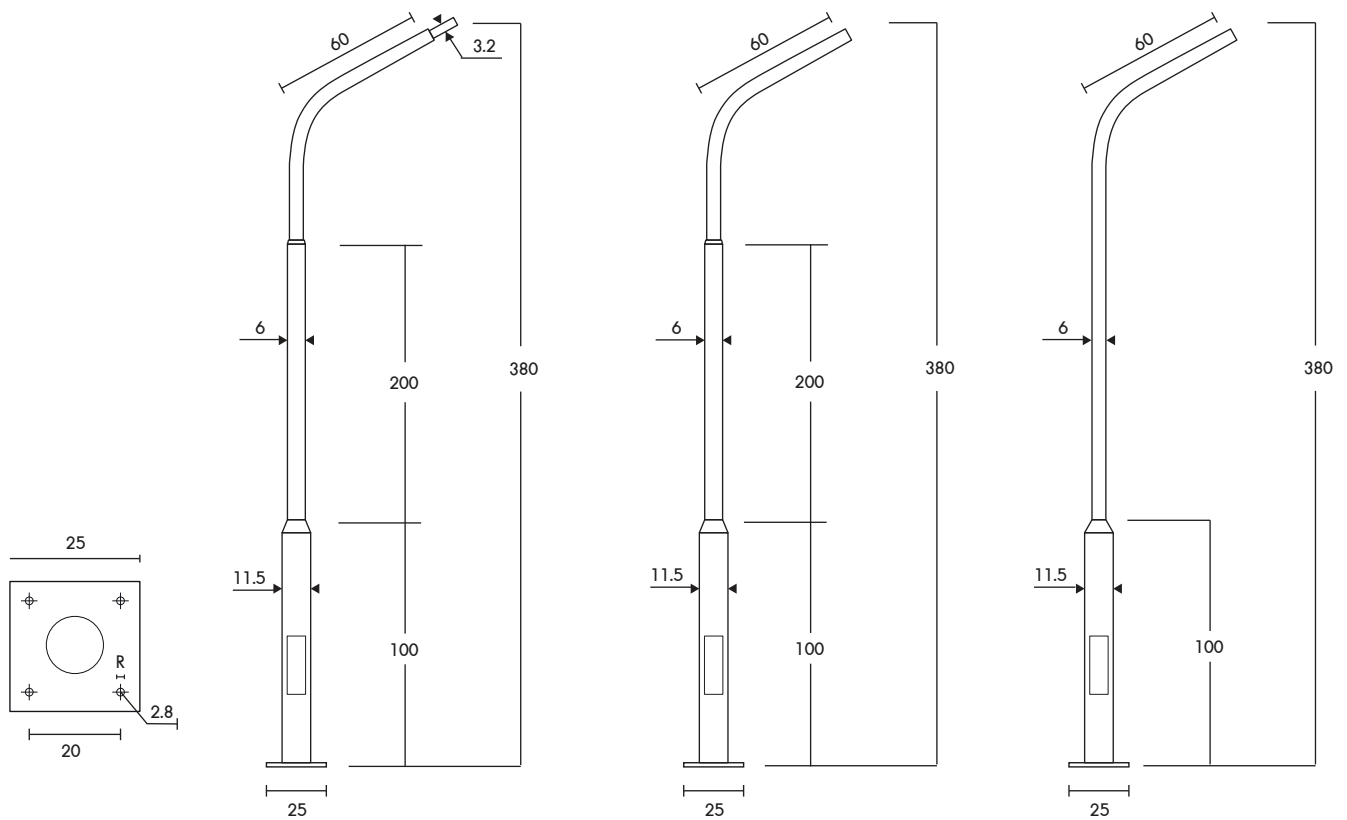
PT-03/4-1/10 ราคา 7,970.- เสาถึงด๊วยปลาย 1.00" สูง 4.00m.
