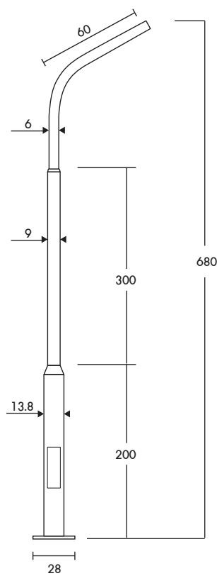
PT-03/7-1/20 ราคา 16,200.- เสาถึงเดี่ยวปลาย 2.00" สูง 7.00m.
