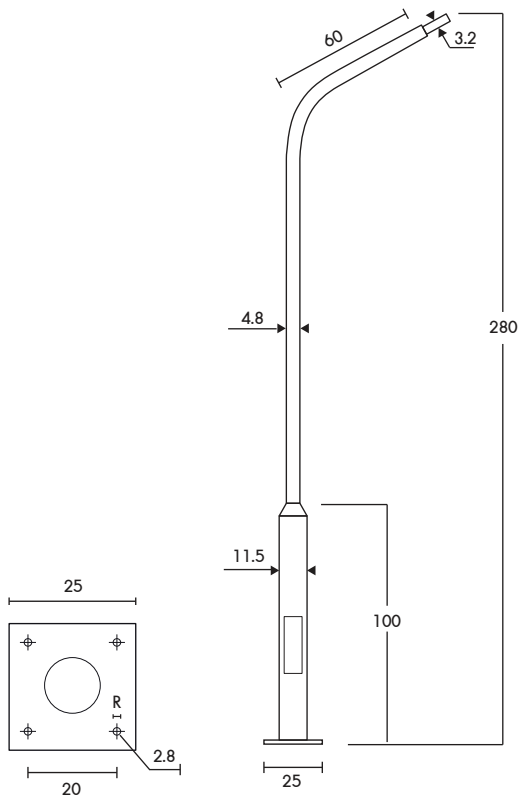
PT-03/3-1/10 ราคา 6,270.- เสาถึงเตี้ยวปลาย 1.00" สูง 3.00m.
