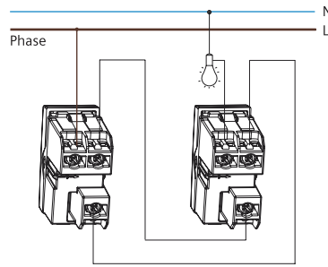
สวิตซ์ 2 ทาง
