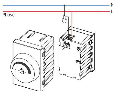
สวิตช์ทรัฟ
