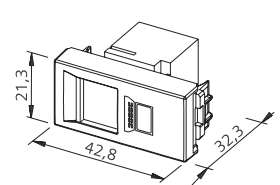
เด้าร์รับคอมพิวเตอร์
