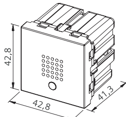
สวิตช์ควบคุมเสียงพร้อมหมตต่อเนื่อง
