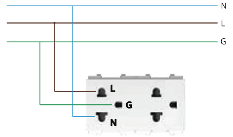
เตารับไฟฟ้า
