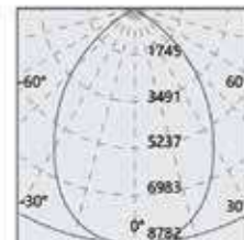
OPL-HB-E150/57-90 150W-5700K-90° 15750LM
