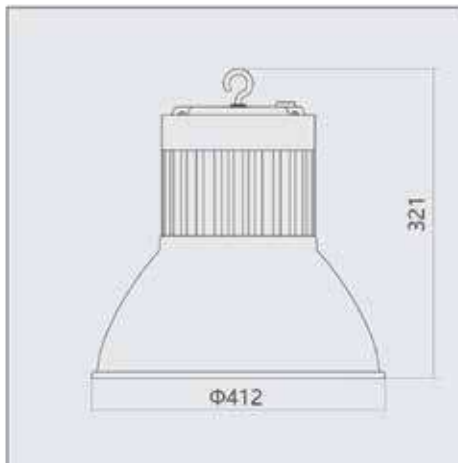
OPL-HB-E150/57-90 150W-5700K-90° 15750LM
