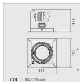
OPL-MATRIX-XL1 / 30 OPL-MATRIX-XL1 / 40 LED 40W (3000K, 4000K)
