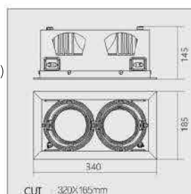
OPL-MATRIX-XL2 / 30 OPL-MATRIX-XL2 / 40 LED 40W x 2 (3000K, 4000K)
