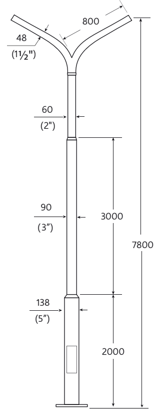
PT-03/8-2/15 เสากิ่งคู่ปลาย 1.50" สูง 8.00 เมตร 16,500.-
