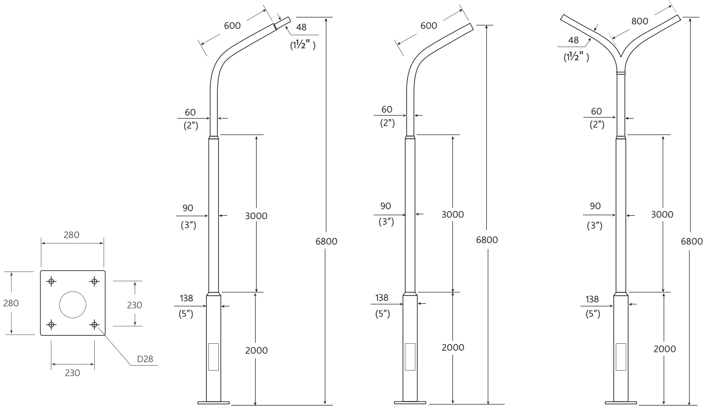
PT-03/7-1/15 เสากึ่งเดี่ยวปลาย 1.50" สูง 7.00 เมตร 14,000.-
