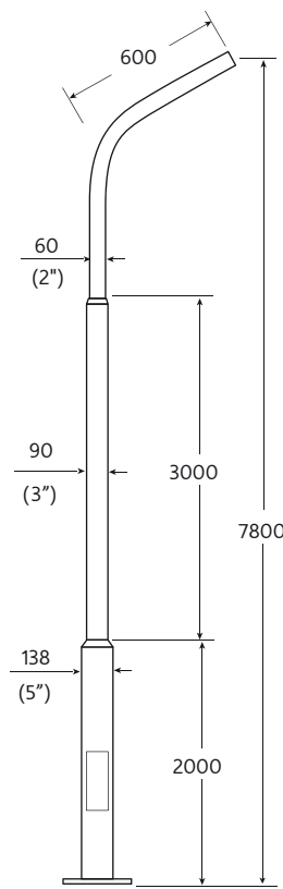
PT-03/8-1/20 เสากิ่งเดี่ยวปลาย 2.00" สูง 8.00 เมตร 15,000.-
