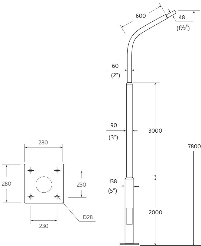
PT-03/8-1/15 เสากิ่งเดี่ยวปลาย 1.50" สูง 8.00 เมตร 15,000.-
