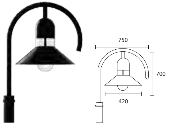
PT-803-3 E27 TORNADO 45W E27 LED A70 14W 10,000.- ( 3m. ) 11,600.- ( 4m. )
