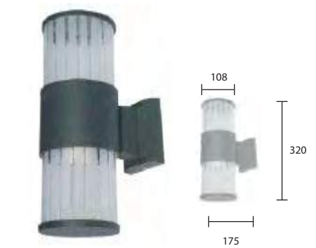
UD-2709/2/BK E27 GENIE 18Wx2 E27 LED A60 7W/9Wx2 1,200.-
