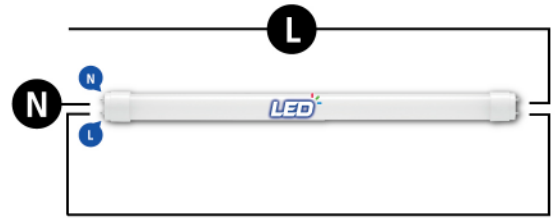
IIUU ไม่มีบัลลาสต์และไม่มีสตาร์ทเตอร์
