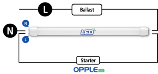
( เปลี่ยนเป็นหลอด LED โดยมีบัลลาสต์เดิม ) IIUU มีบัลลาสต์และสตาร์ทเตอร์
